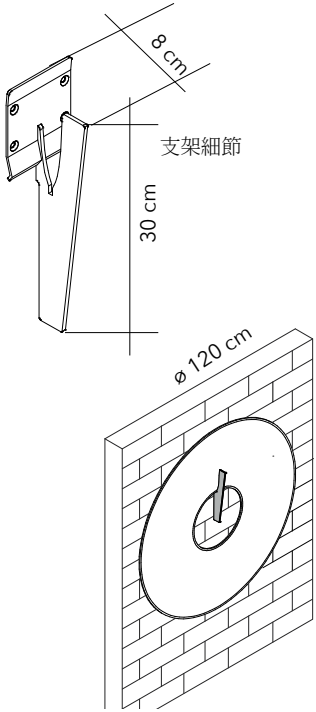
鍍鉻支架
